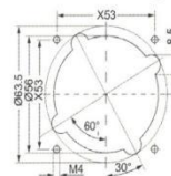
法兰安装尺寸 Assembly dimensions flange socket
