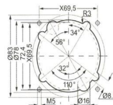
法兰安装尺寸 Assembly dimensions flange socket
