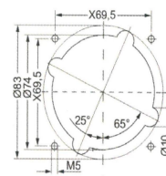
法兰安装尺寸 Assembly dimensions flange socket
