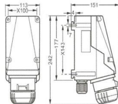
16A 3P 壁式插座 Wall socket 3-pole
