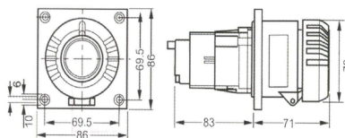
16A 4P 法兰插座 Flange socket 4-pole
