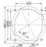
法兰安装尺寸 Assembly dimensions flange socket
