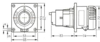
16A 3P 法兰插座 Flange socket 3-pole
